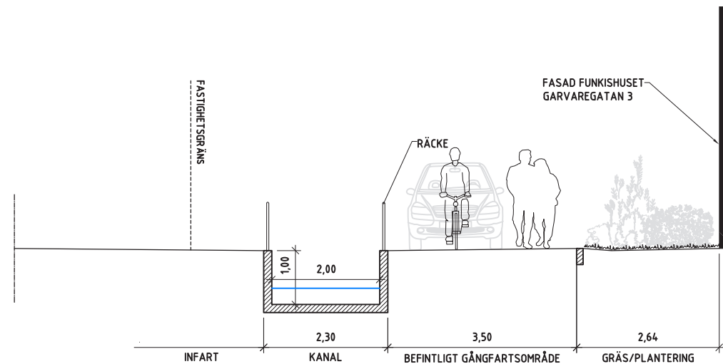
SEKTION B-b SKALA 1:100/A3
