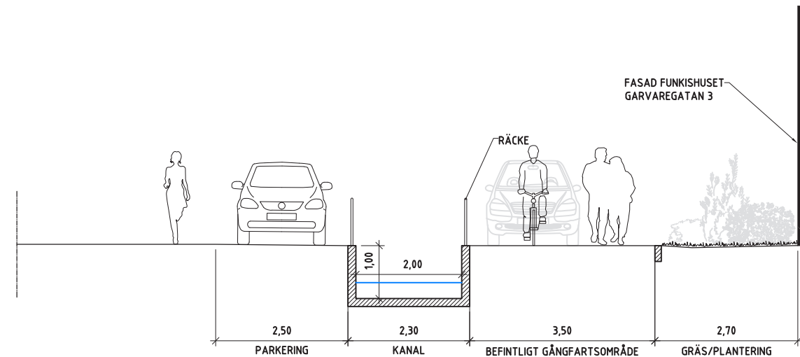
SEKTION A-a SKALA 1:100/A3
