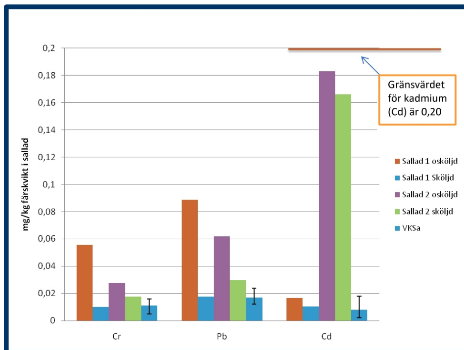
Figur 13. Uppmätta halter av Cr, Pb och Cd i sallad odlade i två trädgårdar i Gusums samhälle. Två samlingsprov (osköljd/sköljd) med 2 dl sallad vardera och per provtagningsplats. VKS anger vanliga metallkoncentrationer i sallad odlade i Sverige (Jorhem & Sundström, 1993). Värdet i denna stapel visar medel-, max- och min-värden för respektive metall.
