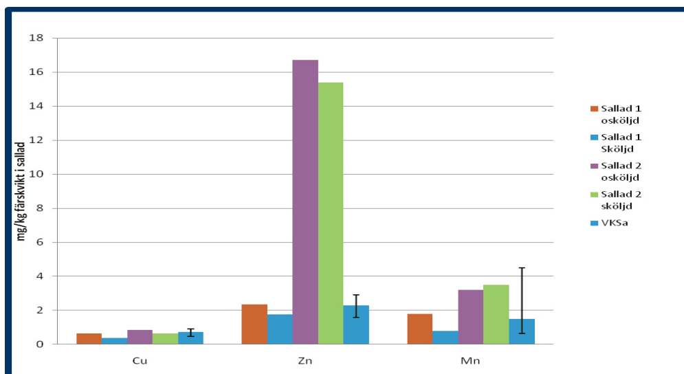
Figur 14. Uppmätta halter av Cu, Zn och Mn, i sallad odlade i två olika trädgårdar i Gusums samhälle. Två samlingsprov (osköljd/sköljd) med 2 dl sallad vardera och per provtagningsplats. VKS anger vanliga metallkoncentrationer i sallad odlade i Sverige (Jorhem & Sundström, 1993). Värdet i denna stapel visar medel-, max- och min-värden för respektive metall.
