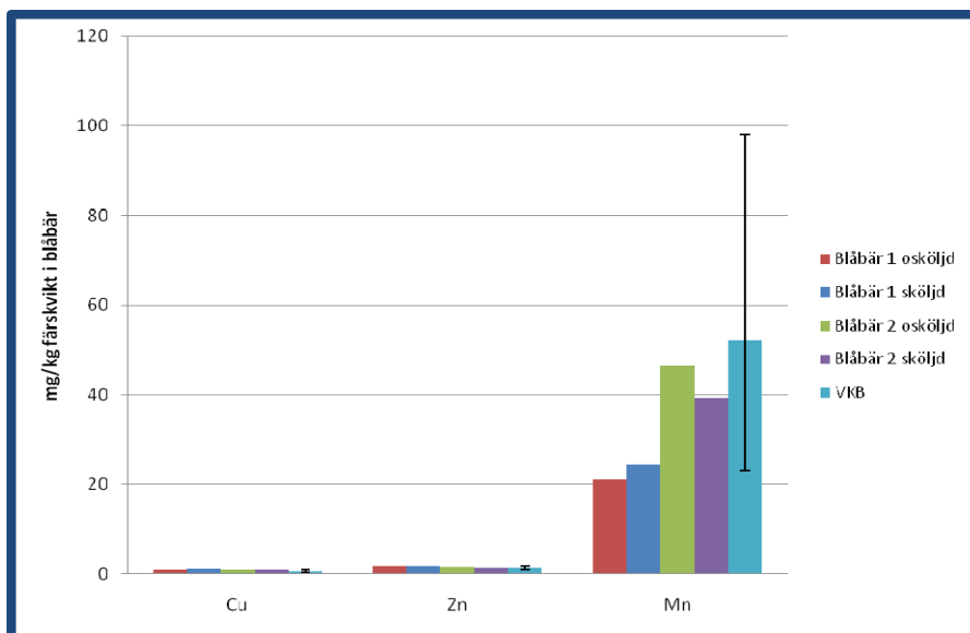
Figur 7. Uppmätta halter av Cu, Zn och Mn i osköljda samt sköljda blåbär plockade vid vattentornet (blåbär 1) och i Dalängsskogen, (blåbär 2) Gusum. Två samlingsprov (osköljd/sköljd) med 3 dl blåbär vardera och per provtagningsplats. VKB anger vanliga metallkoncentrationer i blåbär plockade i Sverige (Jorhem & Sundström, 1993). Värdet i denna stapel visar medel-, max- och min-värden för respektive metall.
