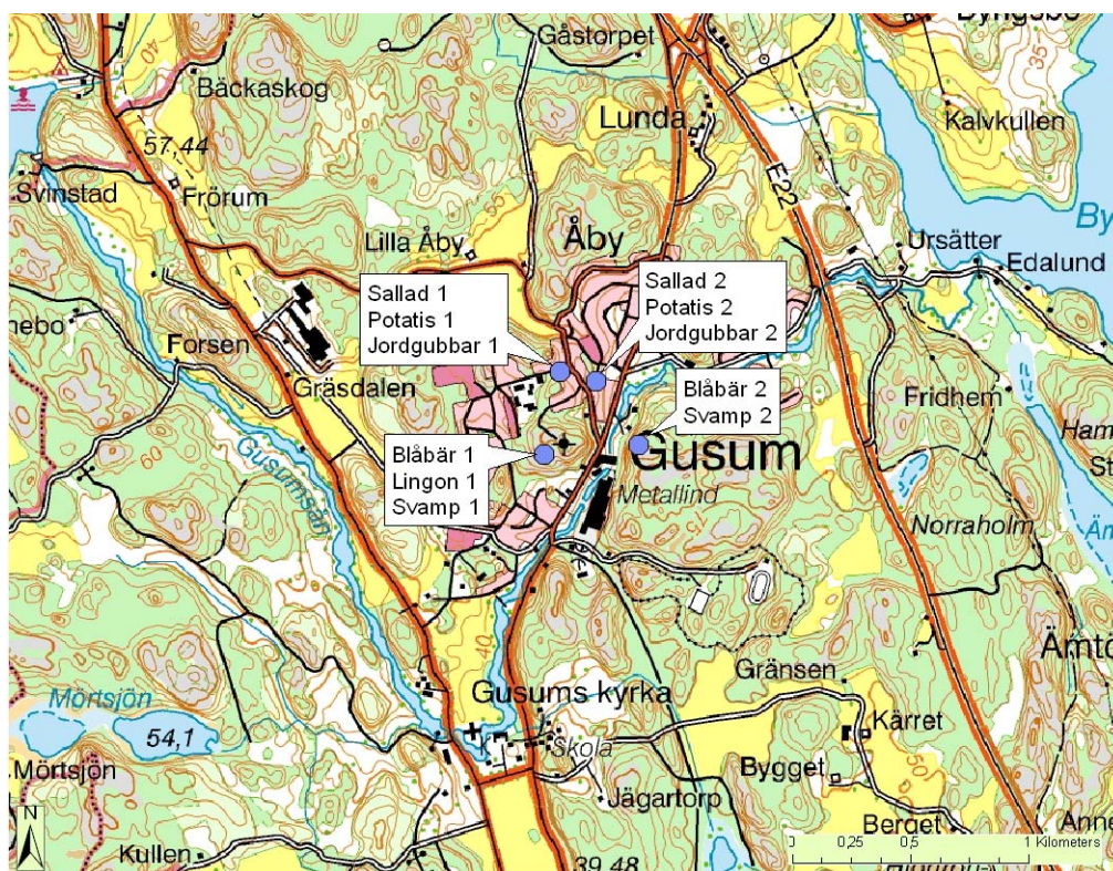
Figur 2. Provtagningsplatser för blåbär, lingon, svamp, sallad, potatis och jordgubbar
