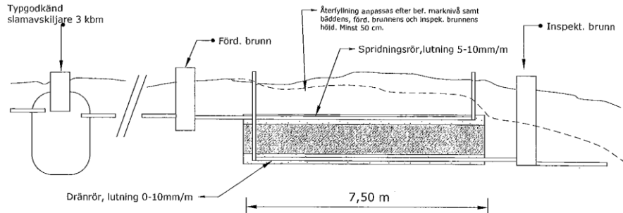
Längdsektion 1:100
