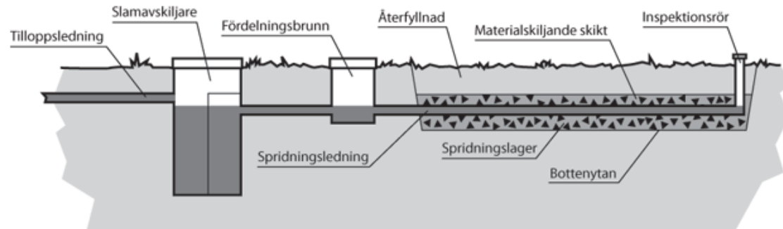
Infiltrationsanläggning
