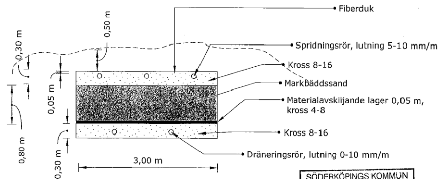
Tvärsektion 1:50
